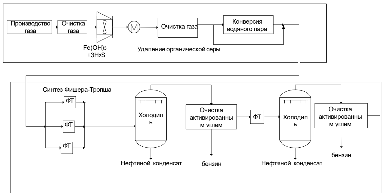
Рисунок 1. Принципиальная схема синтеза Фишера – Тропша при нормальном давлении
